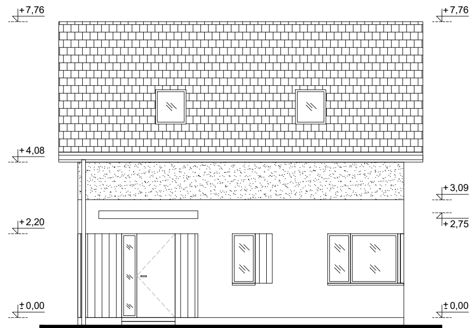
ELEWACJA 4 1:100
