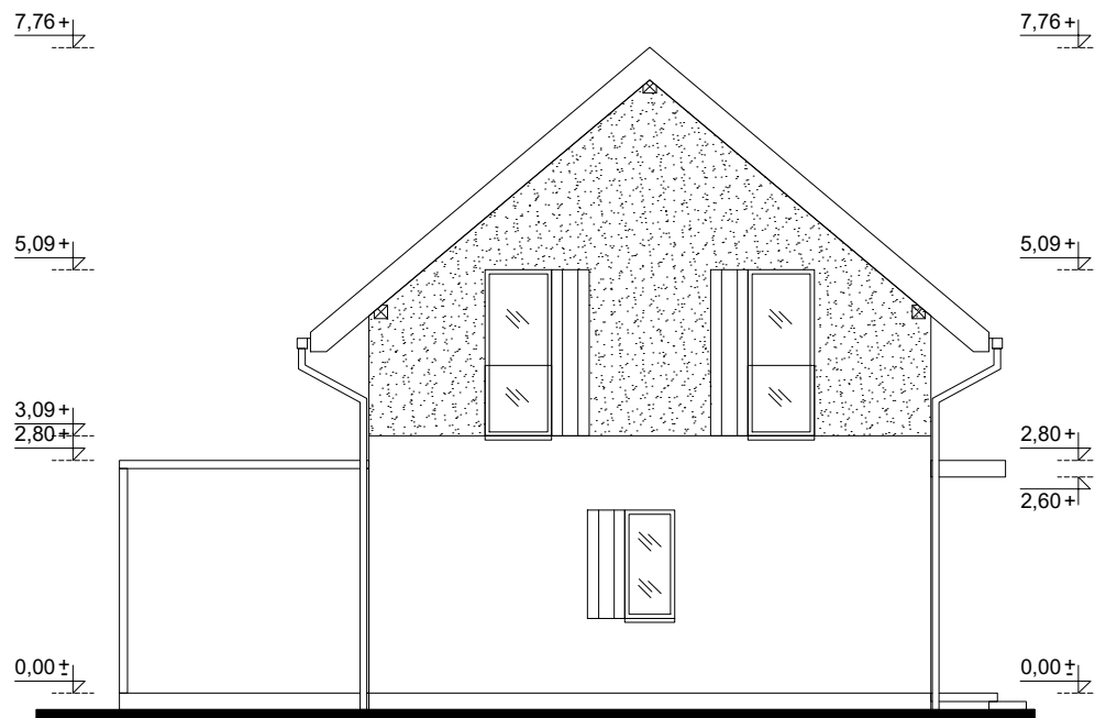
ELEWACJA 1 1:100
