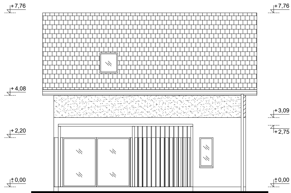
ELEWACJA 2 1:100
